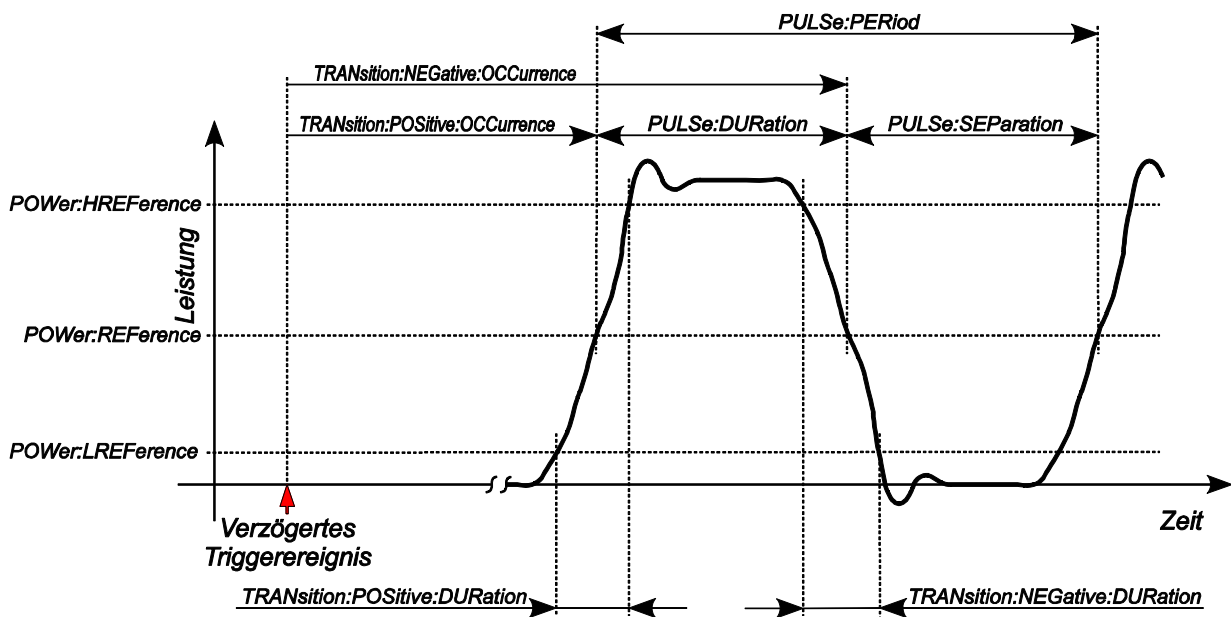
Bild 6-8 Zeitparameter und Referenzpegel eines Traces
